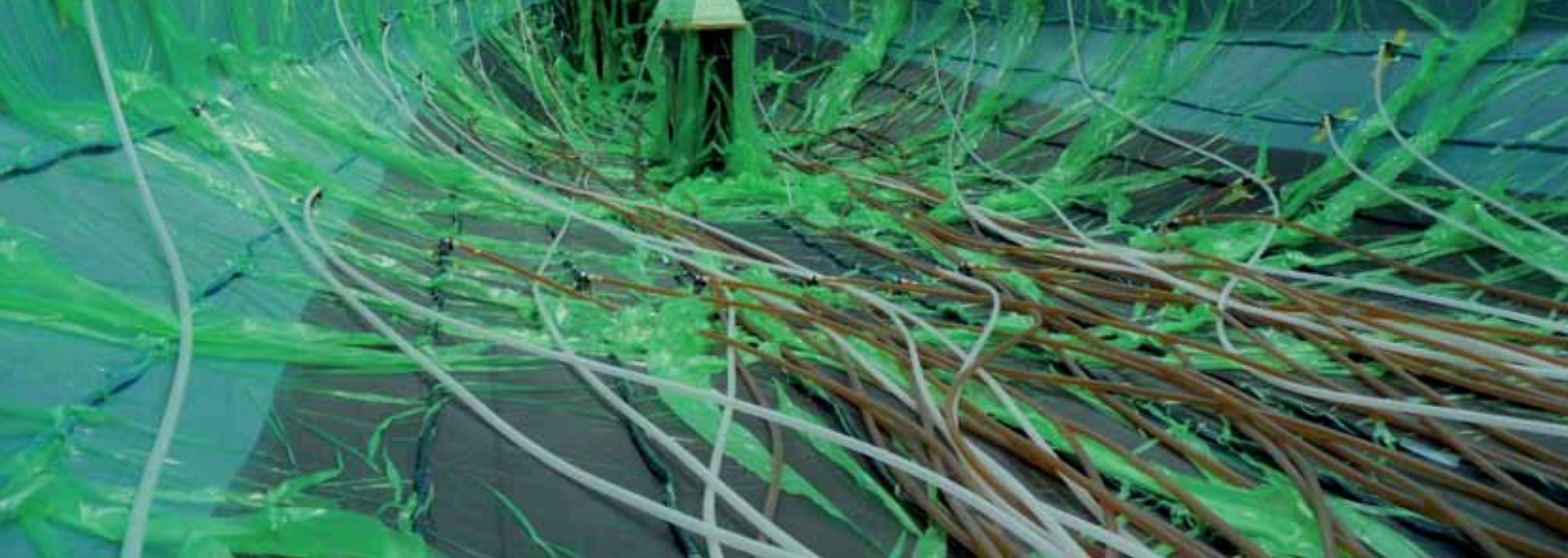
Coque du Pogo 50 en cours d'infusion
