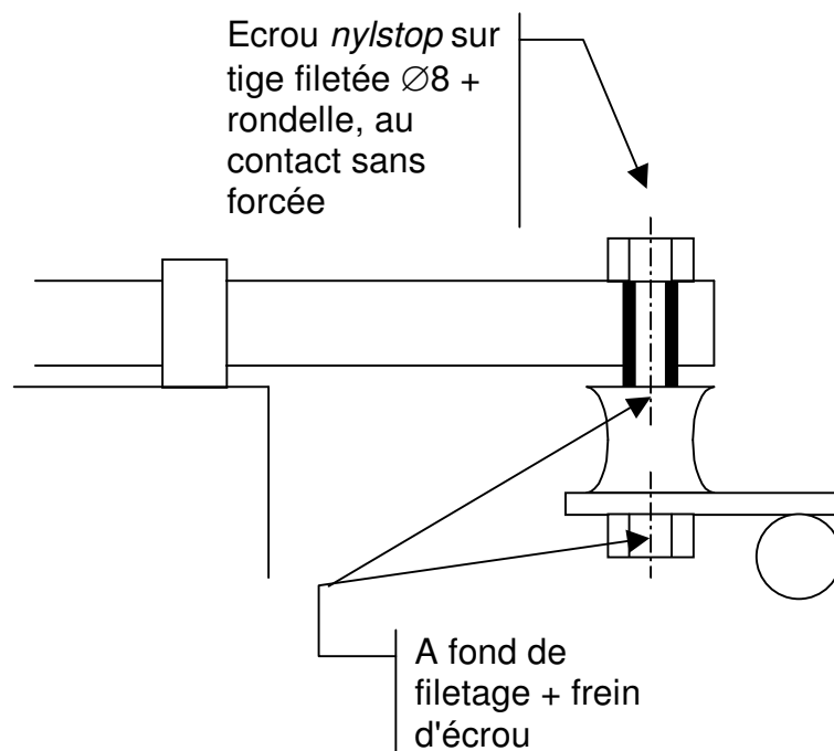
VUE DE COTE
